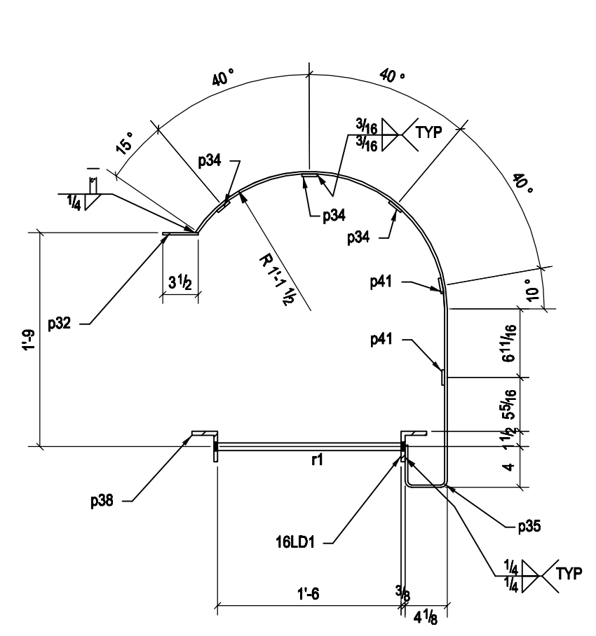
A - A
